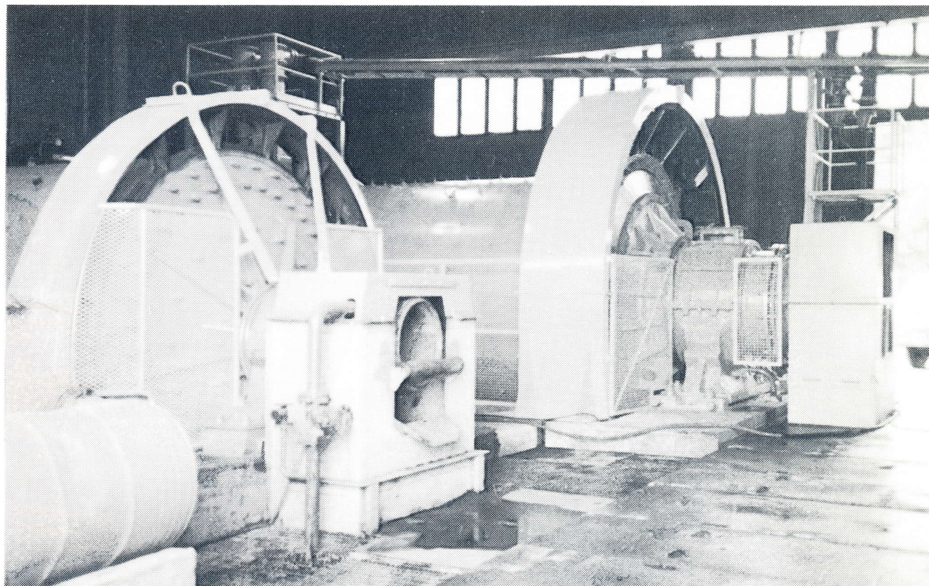
Kuvassa rikastamon jauhatusmyllyjä.
