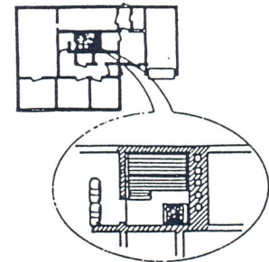
Kellarittomassa omakotitalossa säteilysuojan paikka on talon keskiosassa, mahdollisimman hyvin raskaiden sisäseinien suojassa. Kuvan säteilysuoja on rakennettu talon saunaan. Saunan oven eteen on koottu lisäsuojus hiekkasäkelstä.
