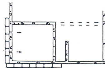
Parhaan suojan antavat pien- ja rivitalojen betonikellarit ja kylmiöt. Maanpinnan yläpuolinen ulkoseinä peitetään esim. hiekkasäkeillä, maa- tai lumivallalla.
