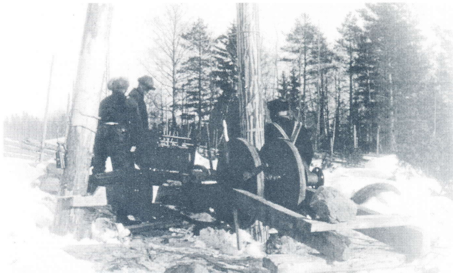
Eristimet vinsataan ylös pylväisiin
