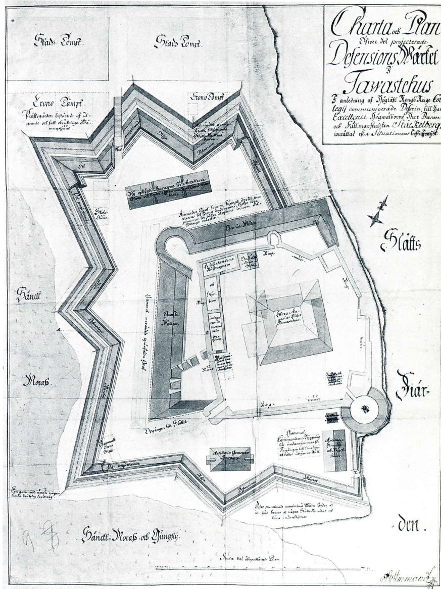
I.G. Ammondin tenjilinnoussuunnitelma vuodelta 1730. Charta och Plan Öfver det projecterade Defensions Wärdet i Tawastehus. Sff. Finland. Tavastehus. Nr. 9. SKA.
