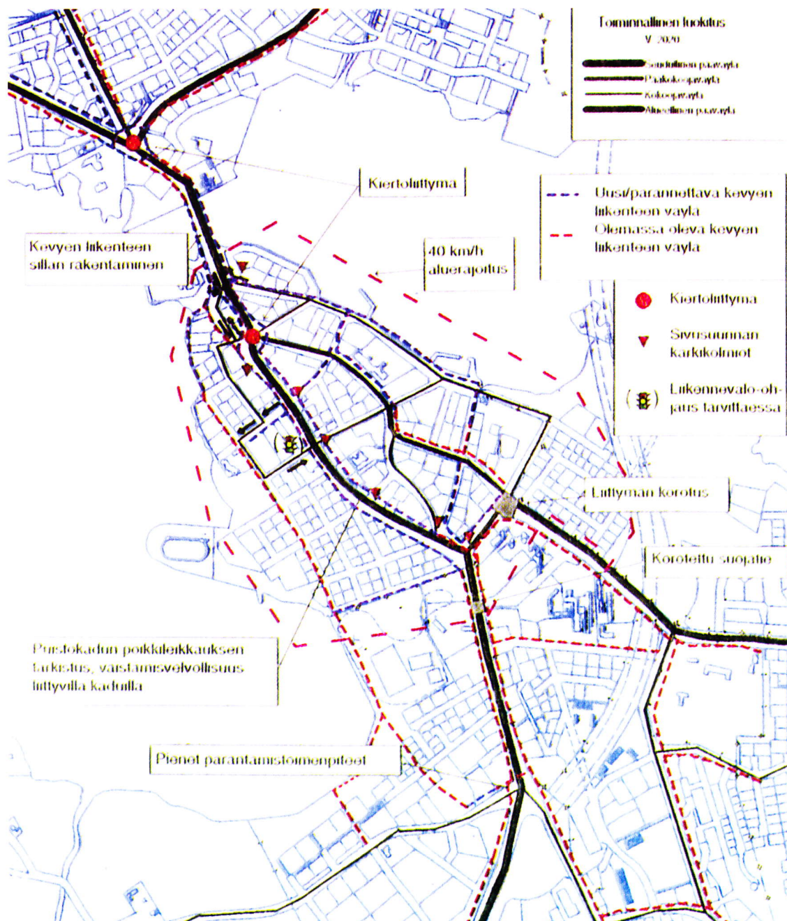
Kuva 12-1. Koko puistokadulla osoitetaan väistämisvelvollisuus liittyyville kaduille. Toimenpiteellä yhdistettynä rakennettaviin hidasteisiin parannetaan liittymien toimivuutta ja turvallisuutta ja ennen kaikkea selkiinnytään nykyisiä epäselviä väistämisvelvollisuuksia.
