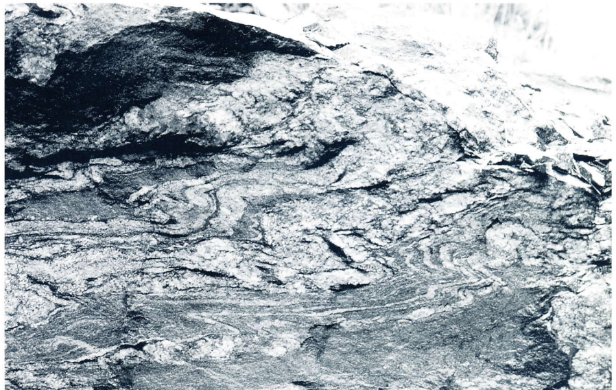
Tampereen–Vammalan ja Hämeelinnan–Someron vulkaanisten kaarten törmäyksessä 1880–1830 miljoonaa vuotta sitten syntyneitä poimurakenteita Velbonkannonmaassa Stormin ja Rämssön välisen tien 2993 varrella olevassa kallioliekkauksessa. Kuva Martti Helin 1999.
